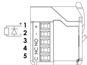
Koblingsskjema uten mikrobryter. Kobling skjer med skruplint.
