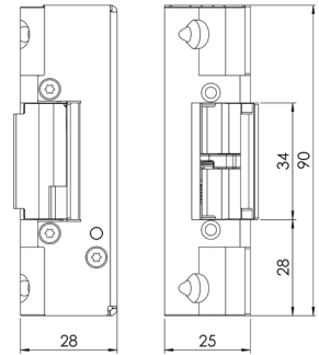
Målsatt tegning STEP 90 Preload.
